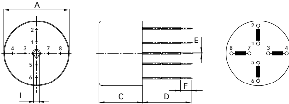
RD 7147, RD 8147
