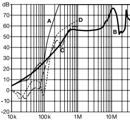
30A types
