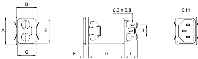
FN 9222ES1
