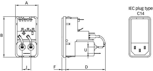
FN 370 / FN 372
