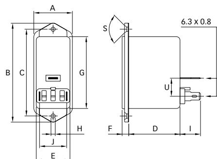
FN 281 / FN 282
