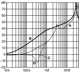
FN 385 / FN 389
