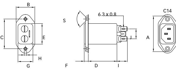
FN 9244U
