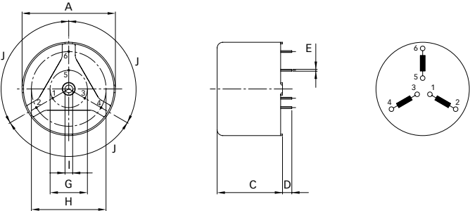
RD 5132
