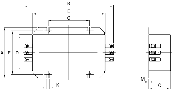
30A types
