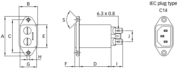
FN 9233E
