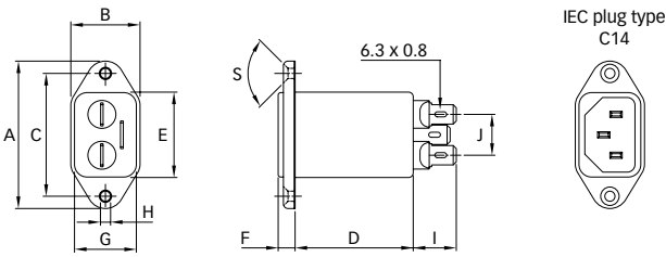
FN 9244E
