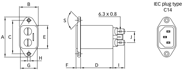
FN 9222E
