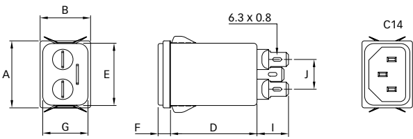
FN 9244ES
