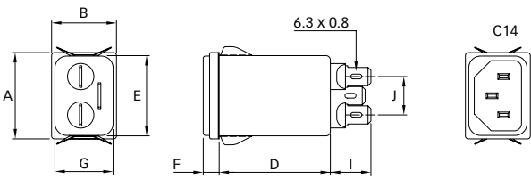
FN 9222ES
