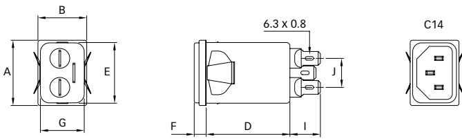
FN 9244ES1
