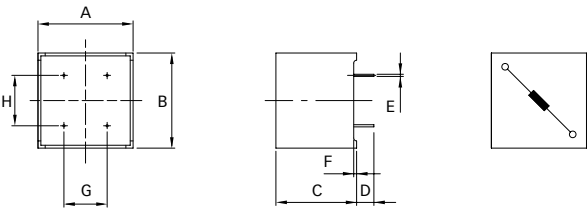
RI 410
