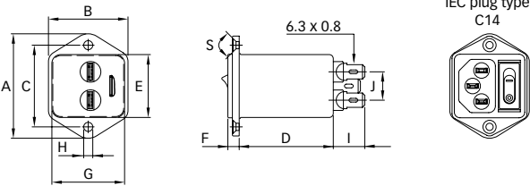
FN 9263S1
